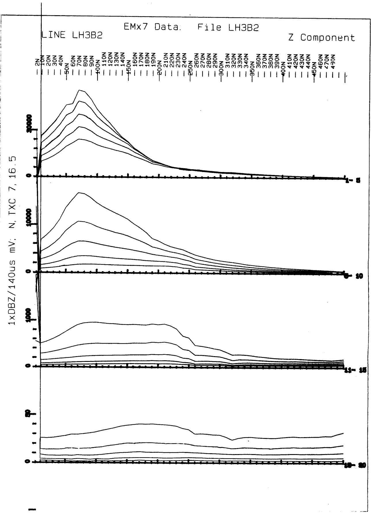
Figura 7.- Registros del sondeo LH-3 con el Bucle 2.
